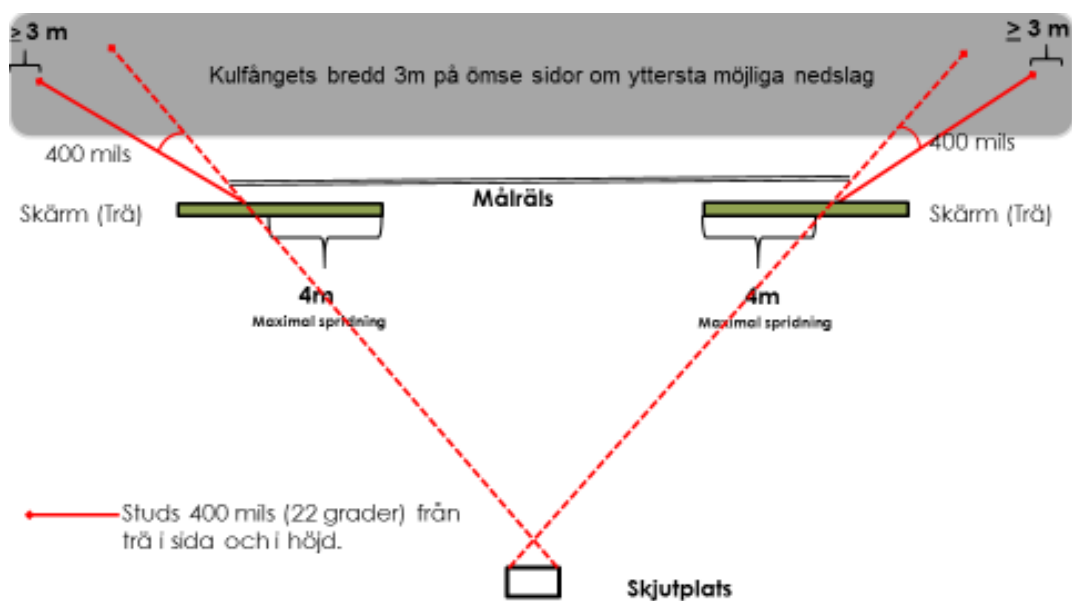
Bild 2:16. Viltmålsbana med genomskjutbar skärm
